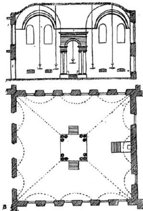
Abb. 37. Grundriss und Schnitt der Maharschalschul
